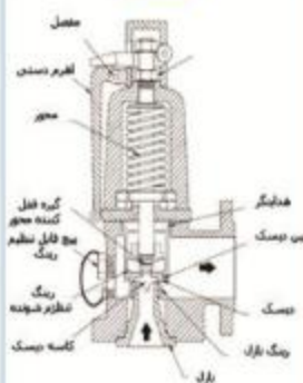
ساختار داخلی یک شیر
