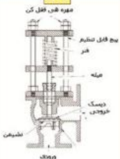
شیر فشار شکن
