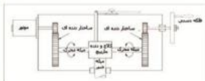
موتور الکتریکی به عنوان فعال کننده شیر به همراه فلکه برآک راه اندازی دستی شیر
