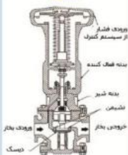
فعال کننده هیدرولیک
