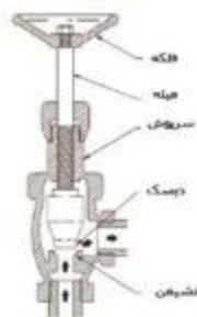
شیر کروی زاویه دار
